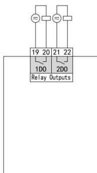
Module-FM3
