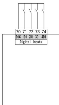
Module-FM2
